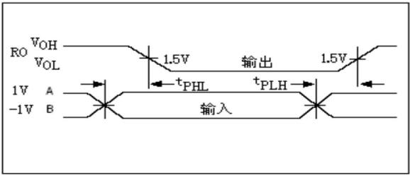
图 8:接收器传播延时
