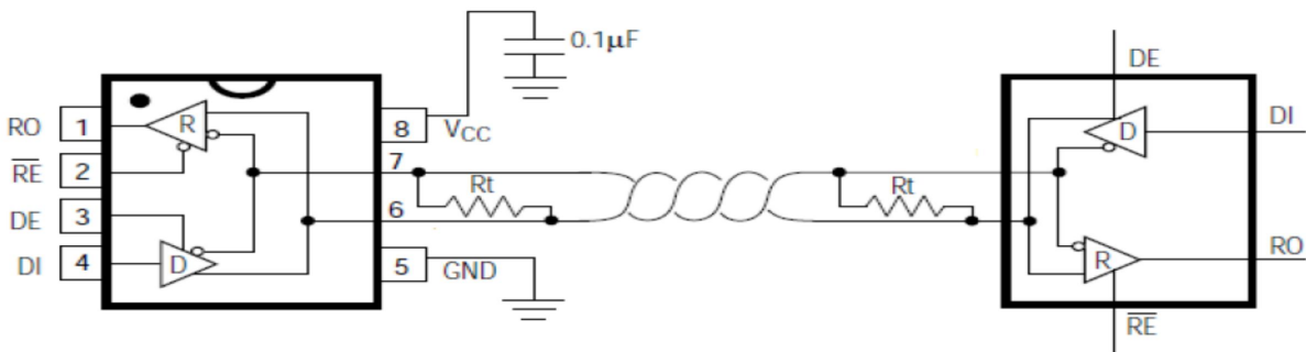
图 1： SP483ECN-TD典型半双工应用电路
