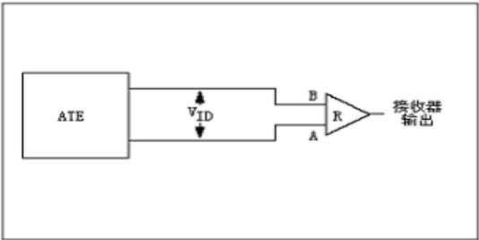
图 10:接收器传播延时测试电路
