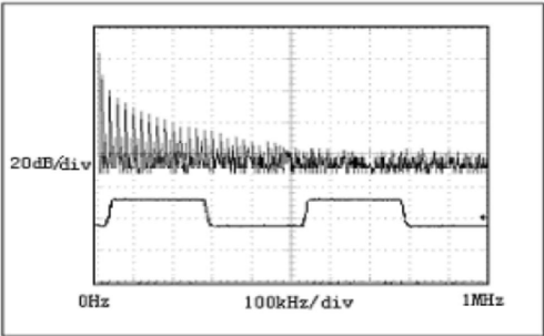
图11: 传输20kHz 信号时SP483ECN-TD驱动器输出波形和FFT图
