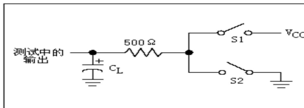
图 5: 驱动器使能/无效定时测试负载
