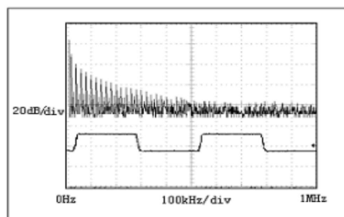
图11: 传输20kHz 信号时SP483CN-TD驱动器输出波形和FFT图
