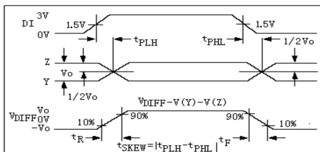
图 6:驱动器传播延时
