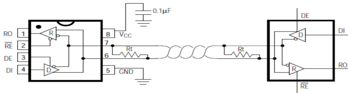
图 1： SP483CN-TD典型半双工应用电路
