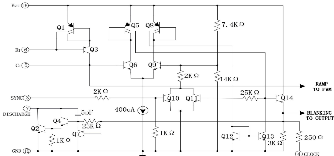
图 c: 振荡器内部电路图
