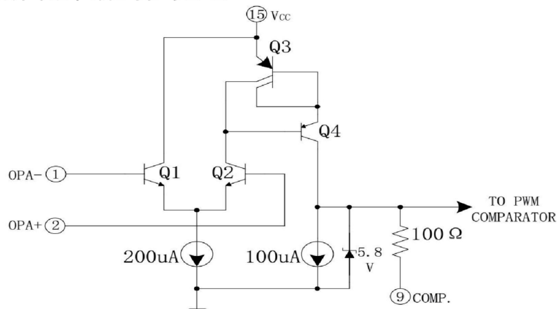
图 a: SG3525 误差放大器内部电路图
