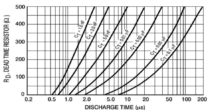
图 e: 振荡器 R_D 和 C_T 对应的放电时间
