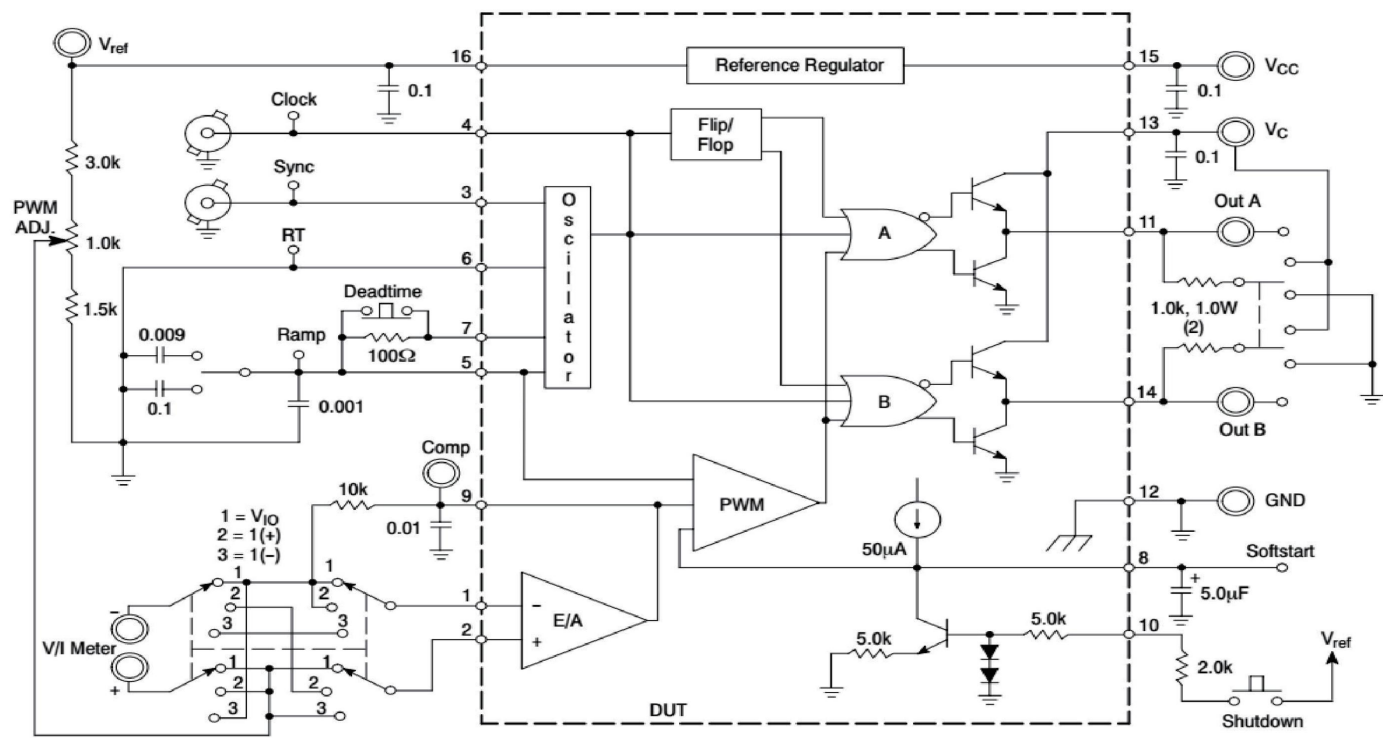
测试性能参数电路图:
