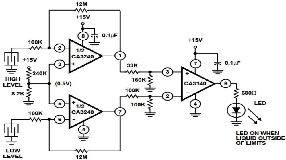
图 2 双电平检测器
