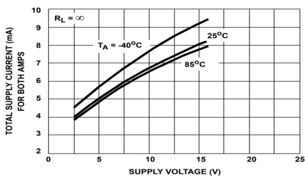
图 8 静态电流 vs 电源电压
