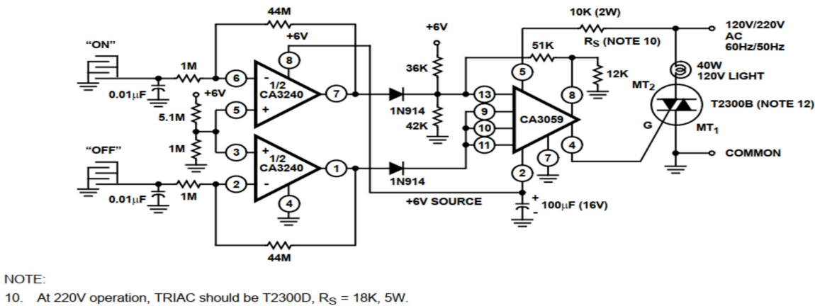
图 1 触摸开关
