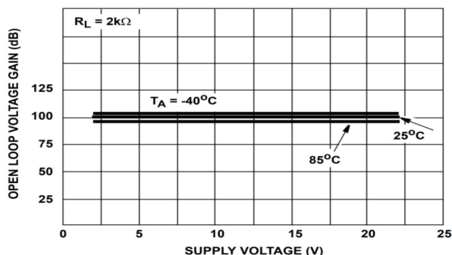
图 5 开路电压增益 vs 电源电压
