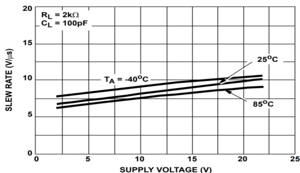
图 7 转换速率 vs 电源电压
