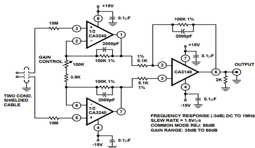
图 4 精密差分放大器
