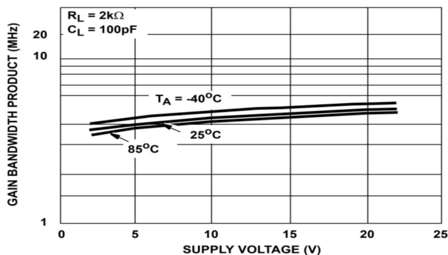
图 6 增益带宽 vs 电源电压
