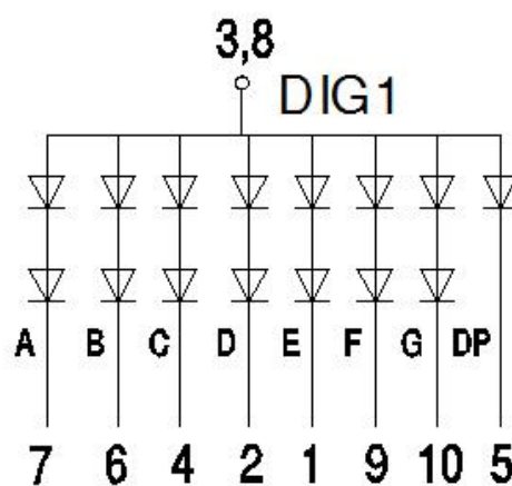
D10016A/B/C/D原理图 共阳
