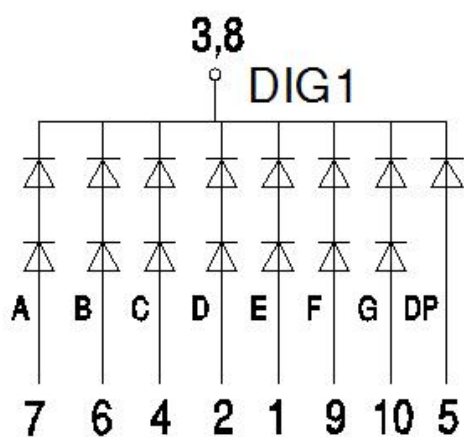
D10016A/B/C/D原理图 共阴
