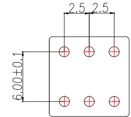
印制线路板 PCB Layout Recommended
