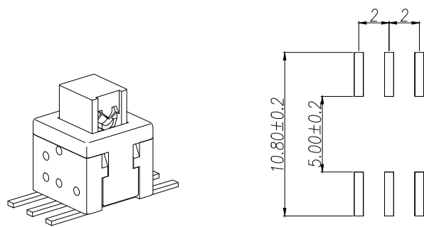
印制线路板 PCB Layout Recommended
