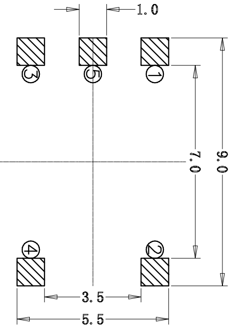
RECOMMENDED P.C.B. LAYOUT 安装尺寸图
