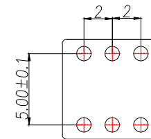
印制线路板 PCB Layout Recommended
