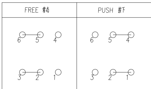
电路图 Circuit Diagram
