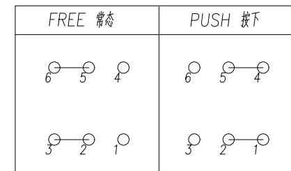
电路图 Circuit Diagram
