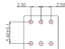
印制线路板 PCB Layout Recommended
