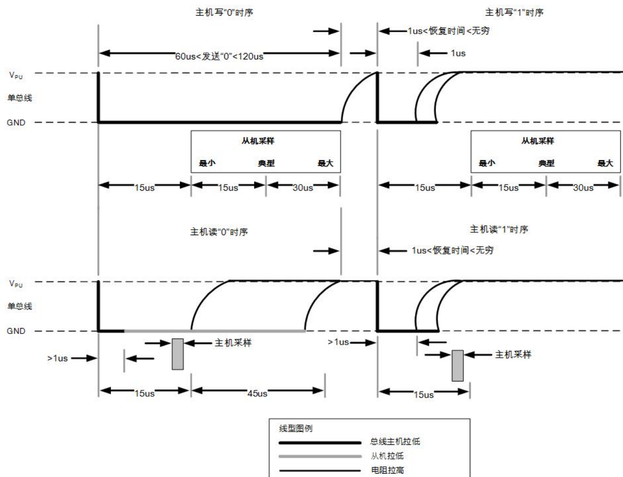
图 11.6-2 读/写时隙时序
