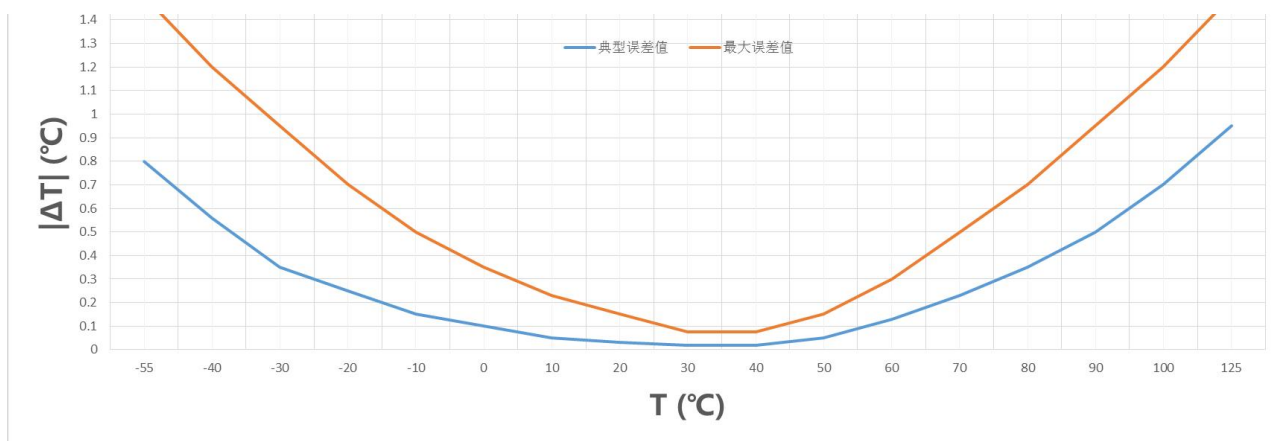
图 7-1 MTS4-OW 精度误差曲线
