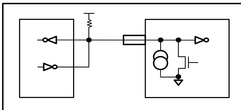
图 11.1 单总线硬件配置
