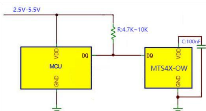
图 9.9-2 寄生模式典型电路图（修改寄存器）
