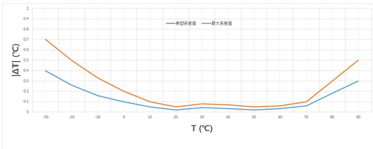
图 7-2 MTS4Z-OW 精度误差曲线
