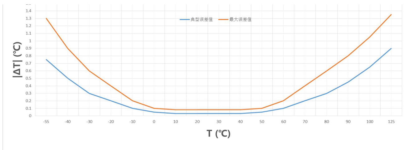
图 7-2 MTS4Z-OW 精度误差曲线
