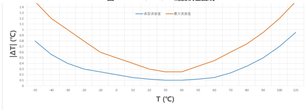
图 7-5 MTS4B-OW 精度误差曲线
