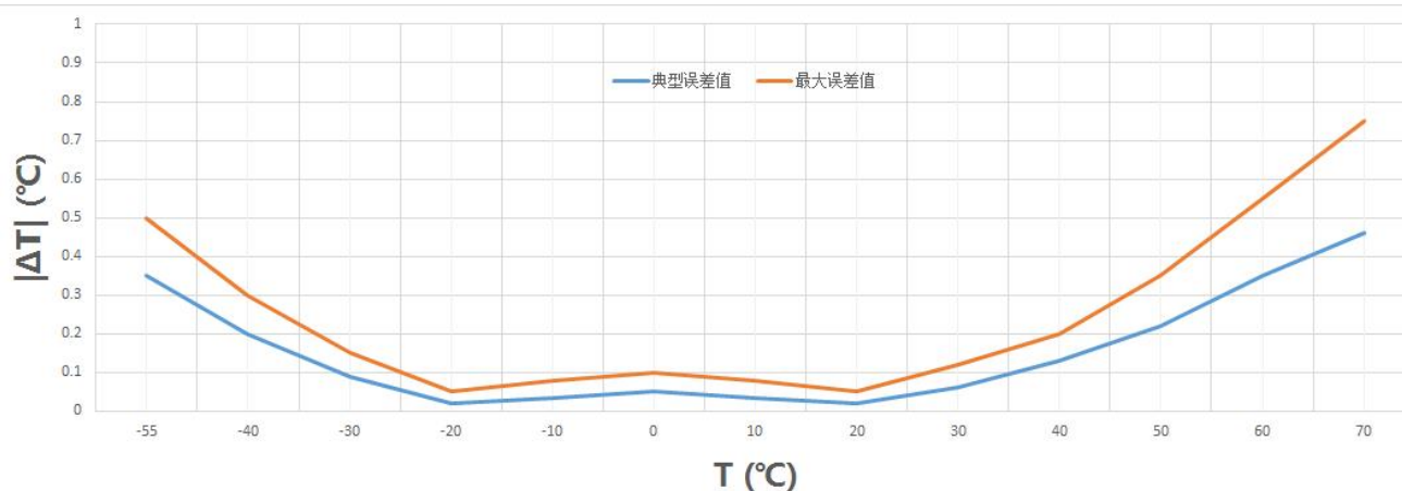
图 7-4 MTS4P-OW 精度误差曲线
