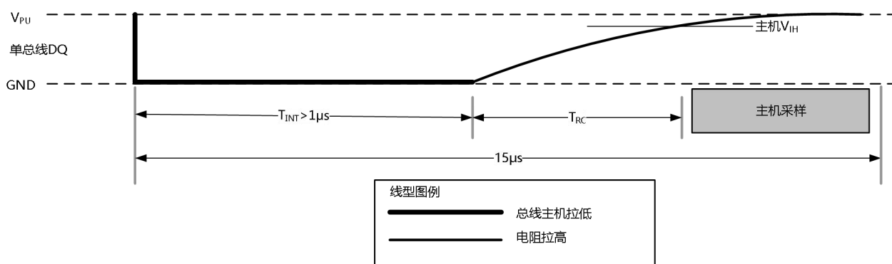
图 11.6-3 详细主机读 1 时序
