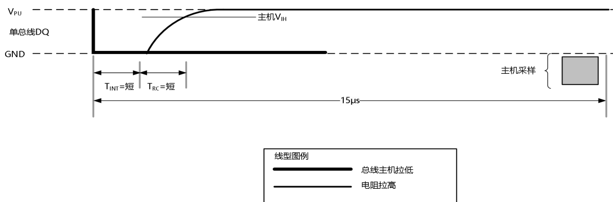
图 11.6-4 推荐的主机读 1 时序
