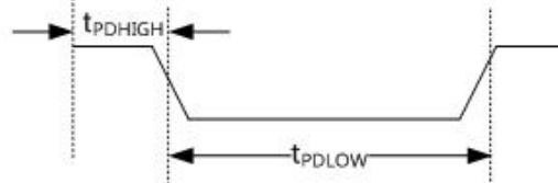
图 11.9 时隙图
