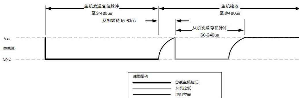
图 11.6-1 初始化时序
