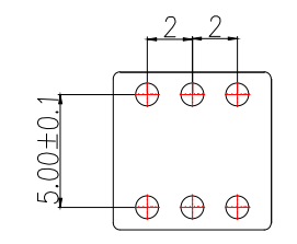
印制线路板 PCB Layout Recommended
