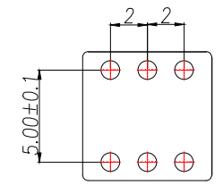
印制线路板 PCB Layout Recommended
