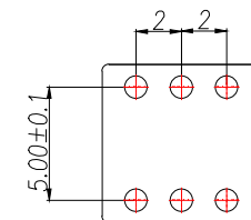
印制线路板 PCB Layout Recommended
