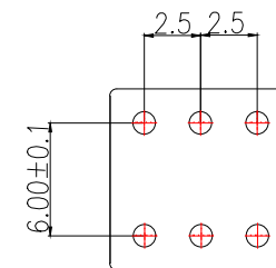
印制线路板 PCB Layout Recommended
