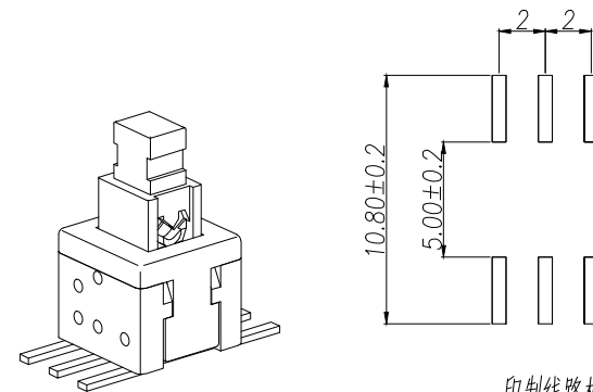
印制线路板 PCB Layout Recommended
