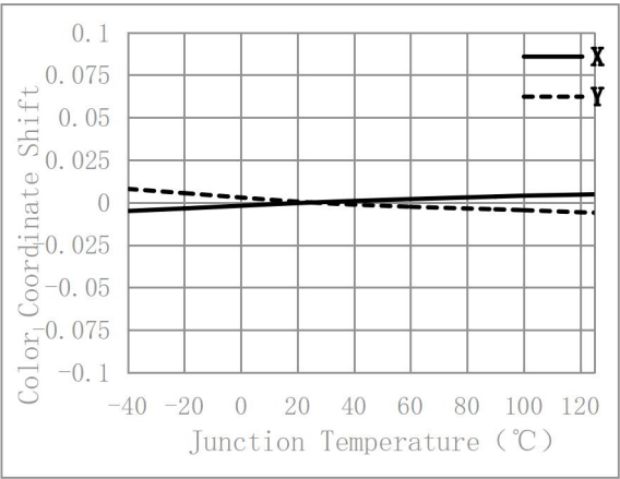
Color coordinate offset(Blue \Delta X 、 \Delta Y )
