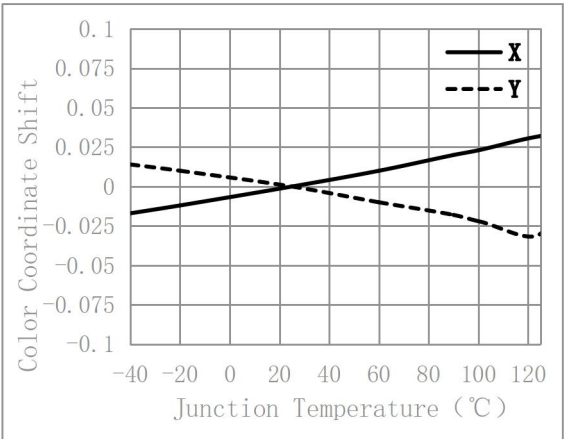
Color coordinate offset(Greed \Delta X 、 \Delta Y )
