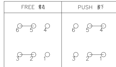
电路图 Circuit Diagram
