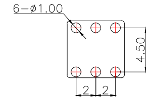
印制线路板 PCB Layout Recommended
