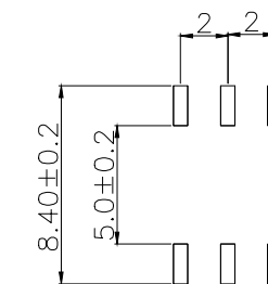
印制线路板 PCB Layout Recommended
