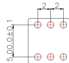
印制线路板 PCB Layout Recommended
