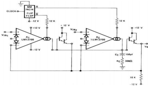
图 21 多路复用器
