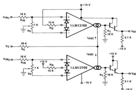
图 15 立体声音频放大器
