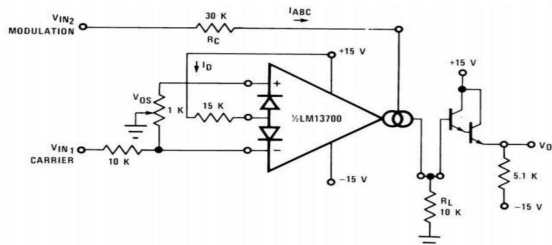
图 19 振幅调制器
