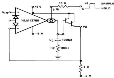
图 23 采样保持电路
