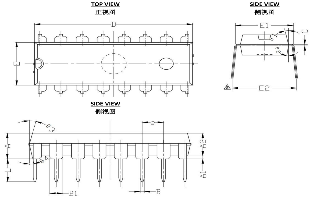
DIP16封装
