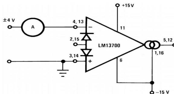
图 26 差分输入电流测试电路
