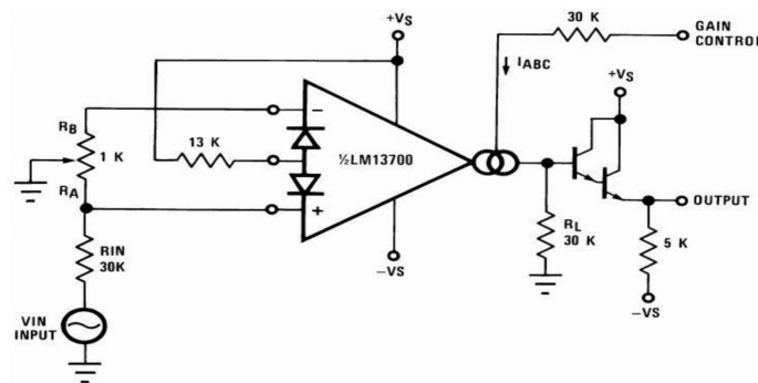
图 10 压控放大器
