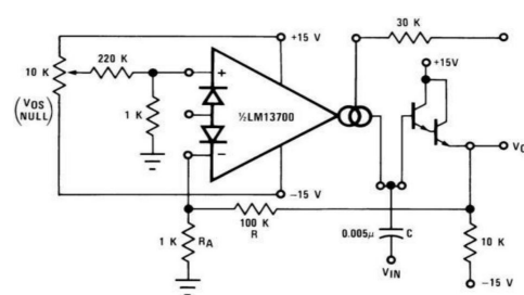
图 18 压控高通滤波器
