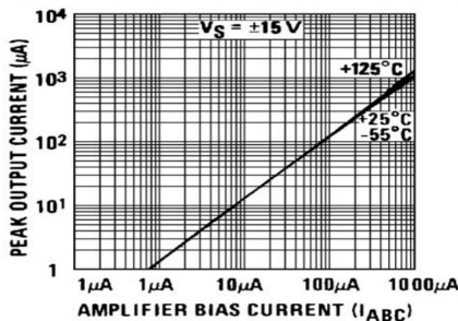
图 4 输出峰值电流与运放偏置电流关系曲线
