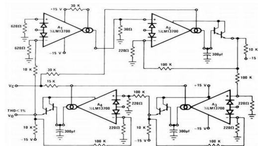
图 16 正弦波压控振荡器
