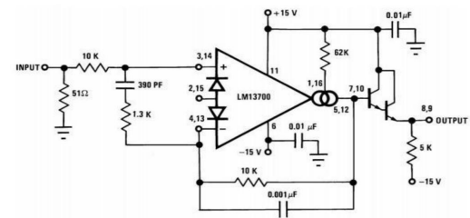
图 24 单位增益跟随
