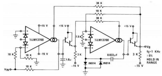
图 22 锁相环
