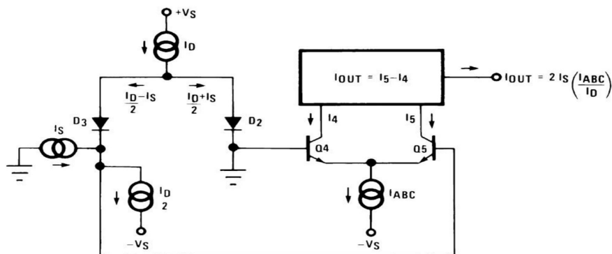
图 12 线性二极管
