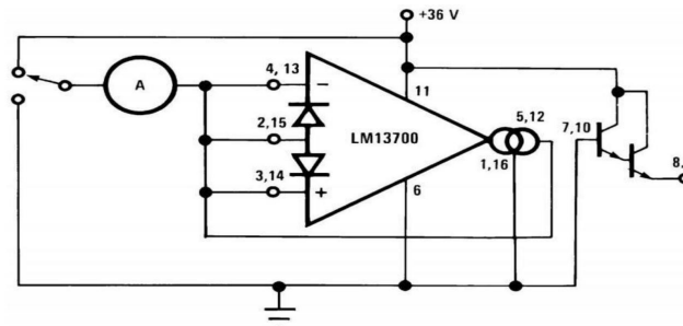
图 25 漏电流测试电路
