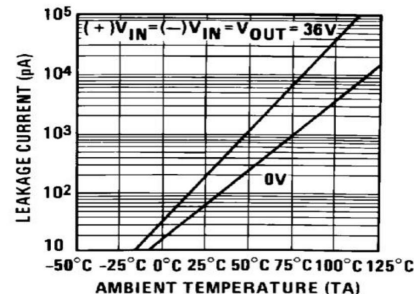
图 5 漏电流与环境温度关系曲线
