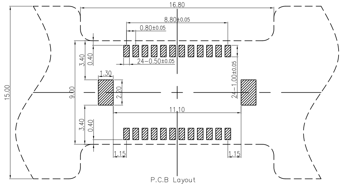
P.C.B Layout
