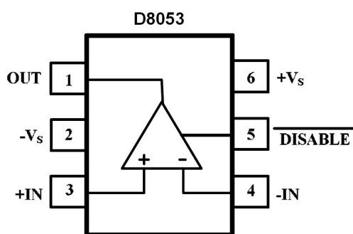
SOT23-6
