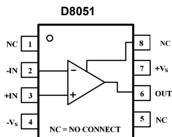
SOP8
