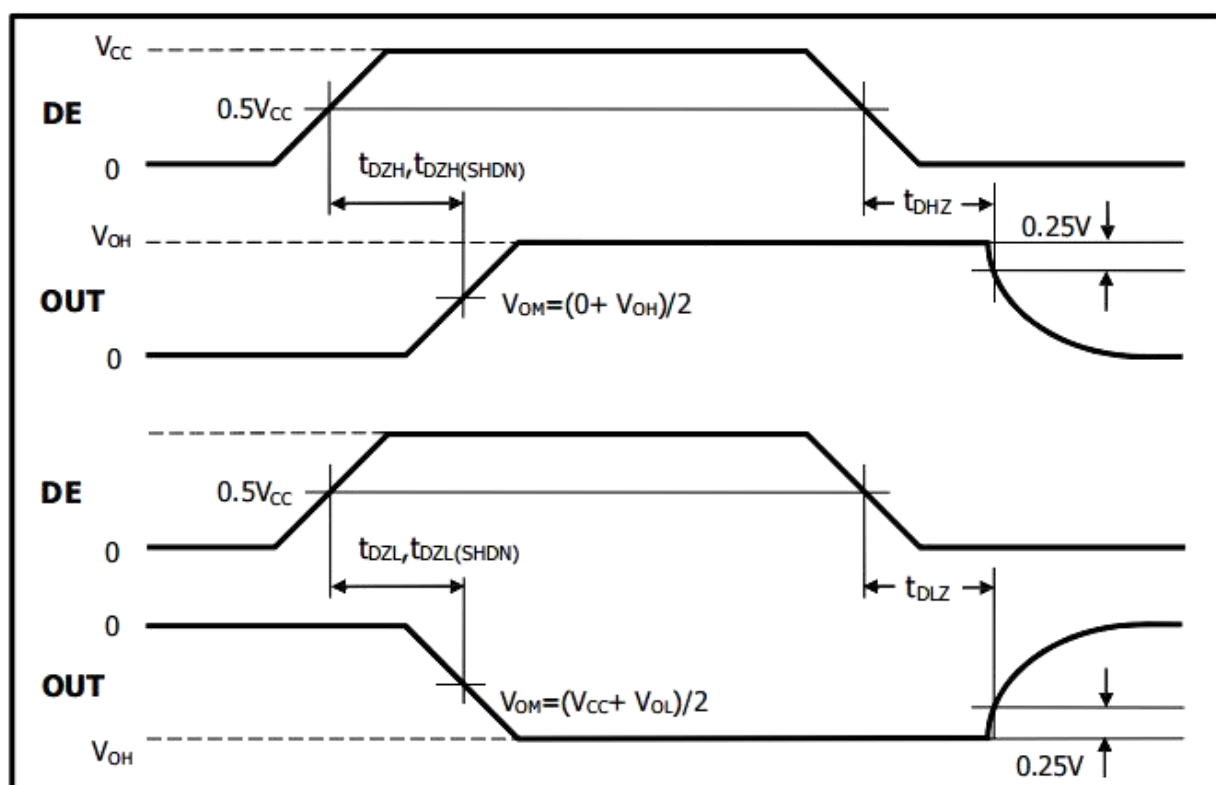
图 5.驱动器传输延时
