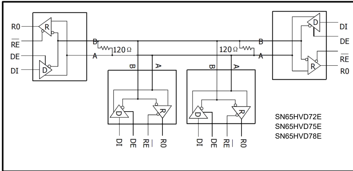
图 11. 典型半双工模式下 RS485 网络
