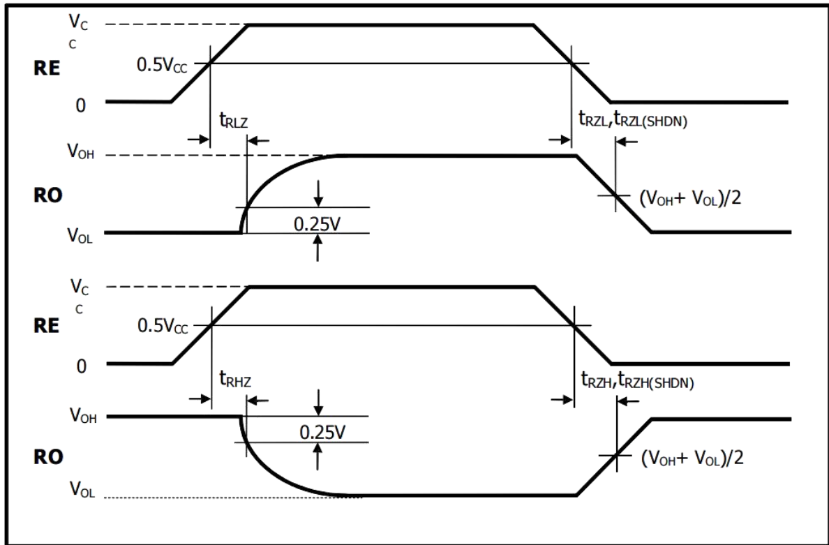
图 9.接收器使能和禁用时序
