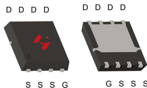
PDFN8L(5x6)
