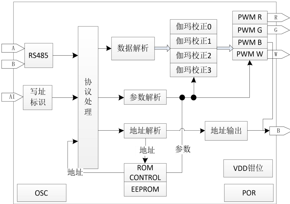
图 8.1 结构框图
