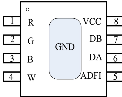
图 5.1 管脚图
