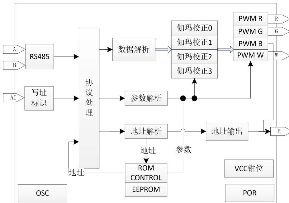
图 7.1 结构框图
