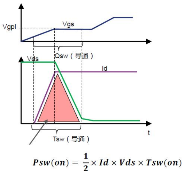
图 11-3 阻性负载条件下的 MOS 开关损耗
