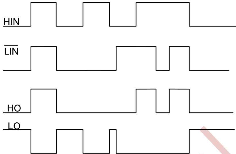
图 9-1 NSG2203U 输入输出时序波形
