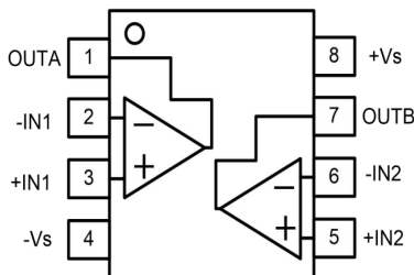
SOP8/MSOP8/TSSOP8
