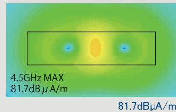
DF40GT
