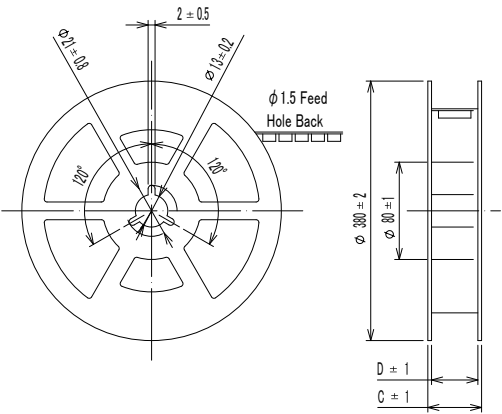
Reel Dimensions
