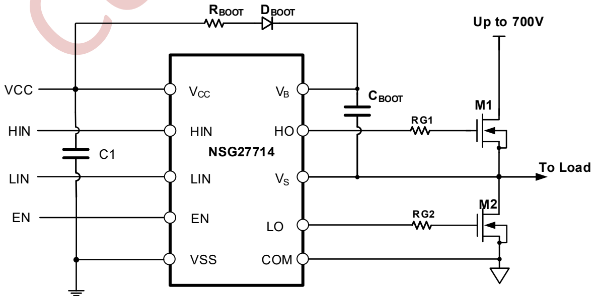
图 11-2 典型应用电路图
