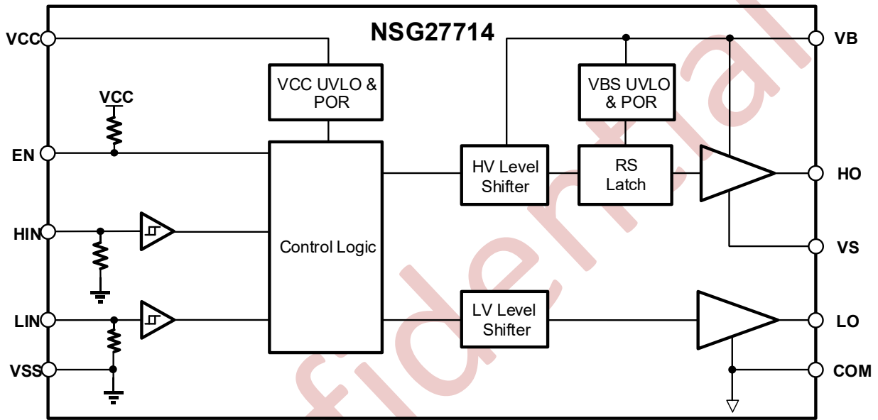
图 11-1 NSG27714 功能框图
