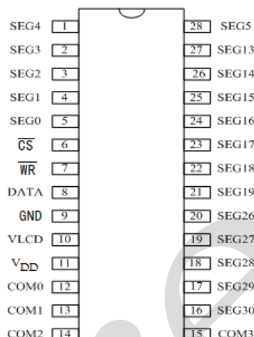
SOP28
