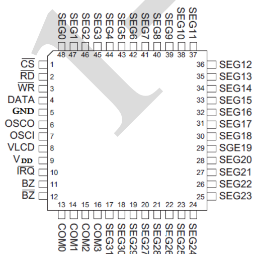
LQFP48
