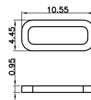
防水圈图示
