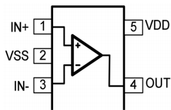
SOT23-5/SC70-5
