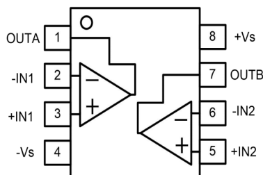
SOP8/MSOP8
