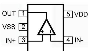
SOT23/SC70
