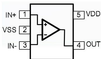
SOT23/SC70
