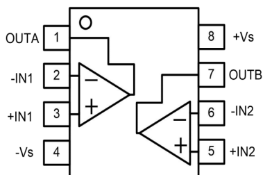
SOP8/MSOP8/TSSOP8
