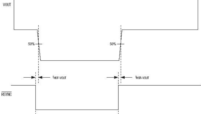
图9. VOUT和HSYNC行同步时序(NTSC和PAL, 内同步模式)
