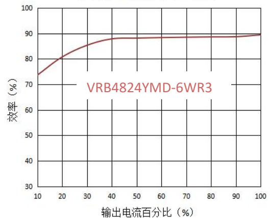
输出效率vs输出负载 (48V输入)
