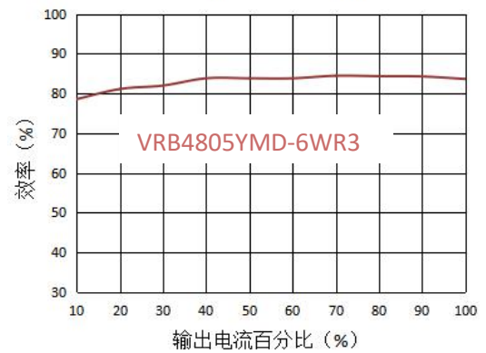
输出效率vs输出负载 (48V输入)
