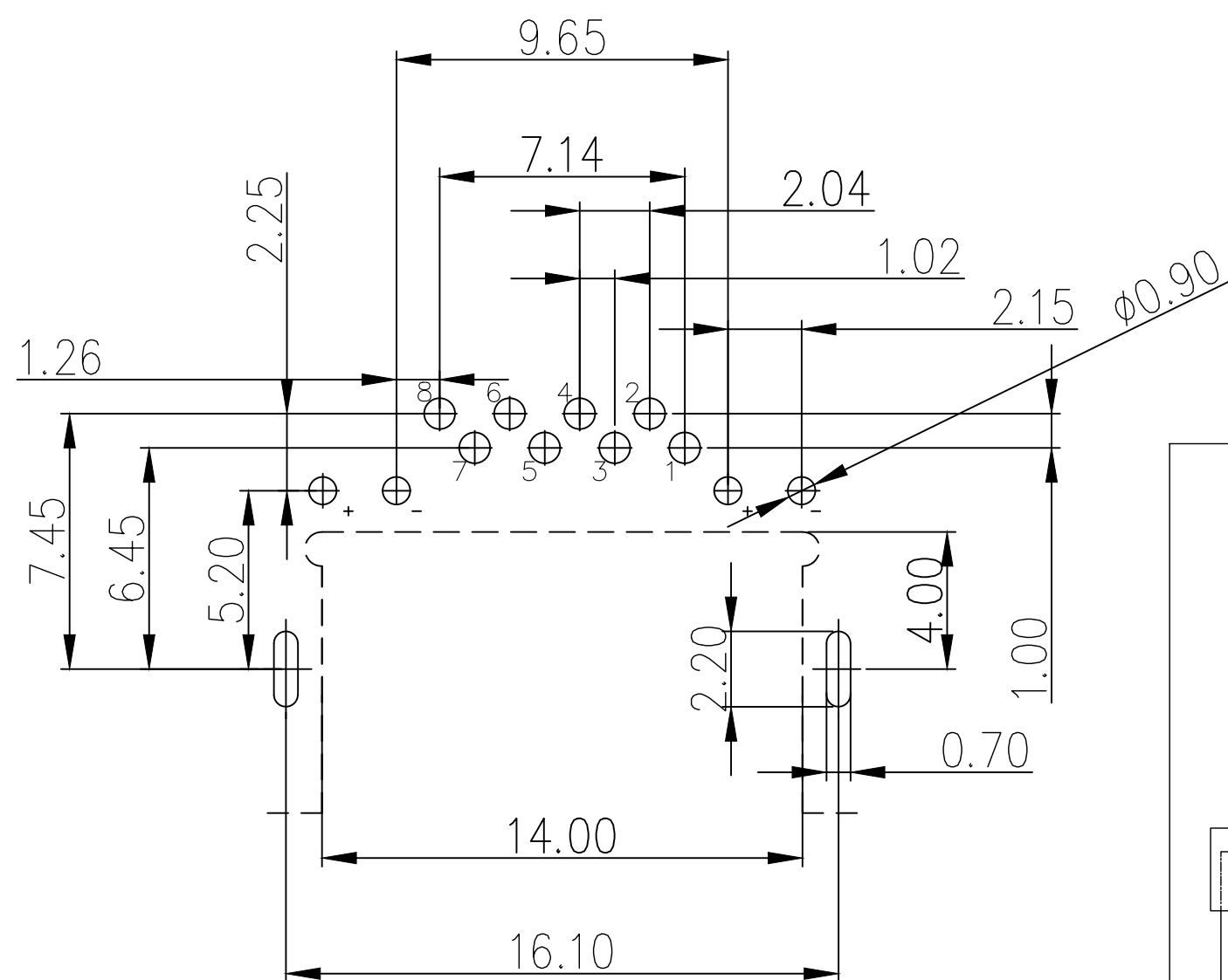
PCB 参考图
