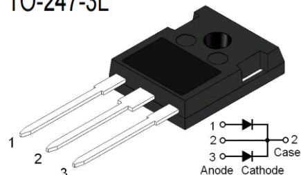
TO-247-3L
