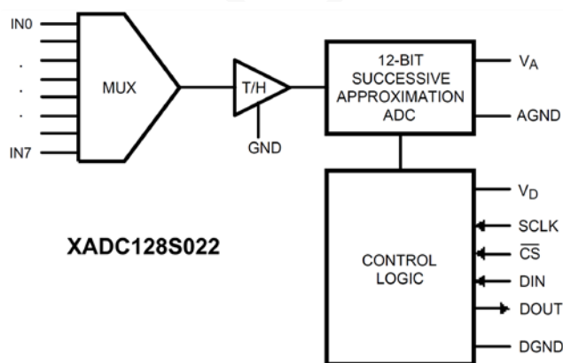
原理图
