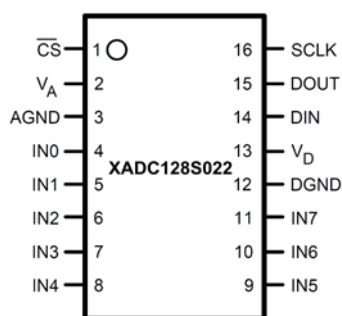
引脚图
