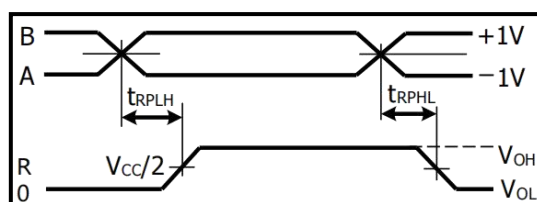
图 8.接收器传输延时
