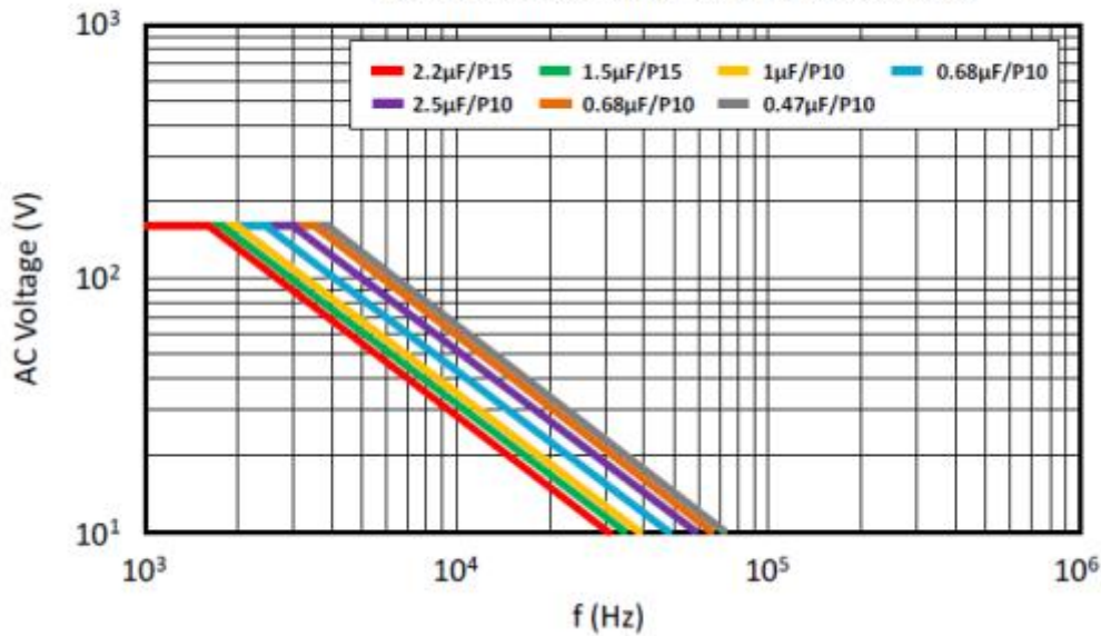
小型化CBB21B(M) 450VDC/160VAC
