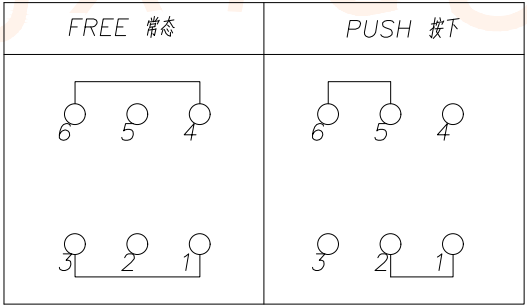
电路图 Circuit Diagram
