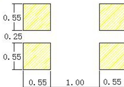
建议焊盘尺寸
