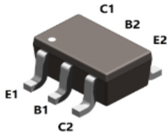
SOT-363
