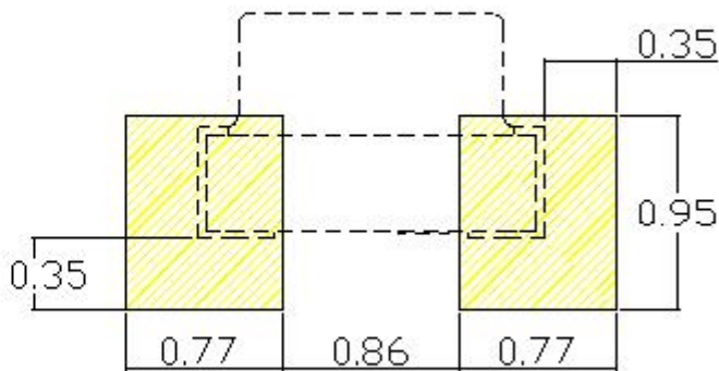
建议焊盘尺寸
