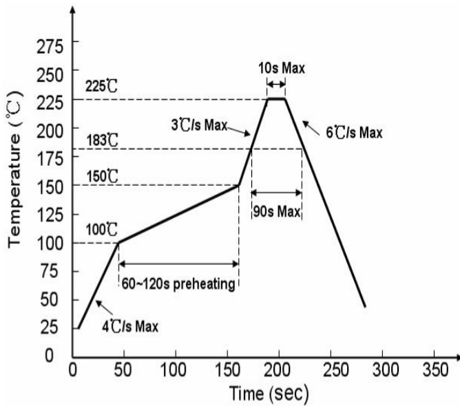
有铅制程
