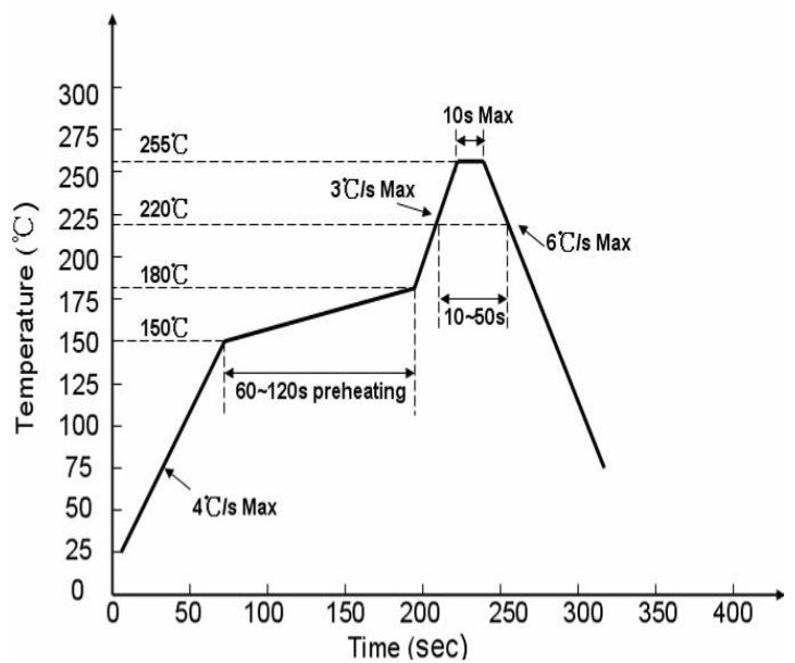
无铅制程
