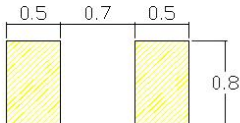
建议焊盘尺寸
