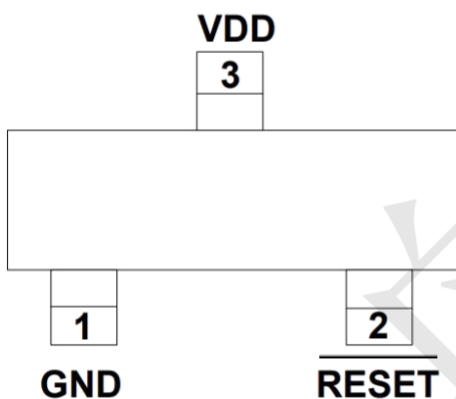
SOT23
